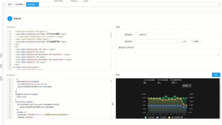
图 5-6 自定义组件
